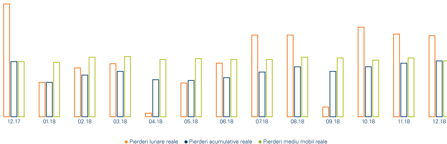
Evoluția pierderilor de energie electrică, 2018
